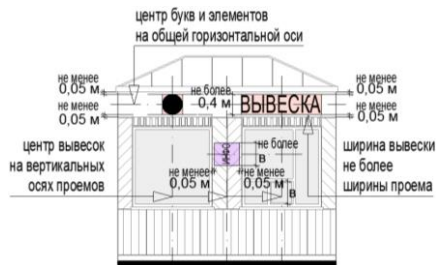
главный фасад:
